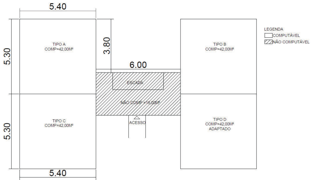
BLOCO A PAVIMENTO TÉRREO ESC: 1/100
