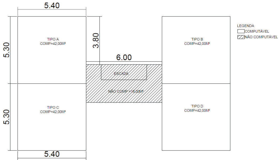
BLOCO A PAVIMENTO TIPO X 4 ESC: 1/100
